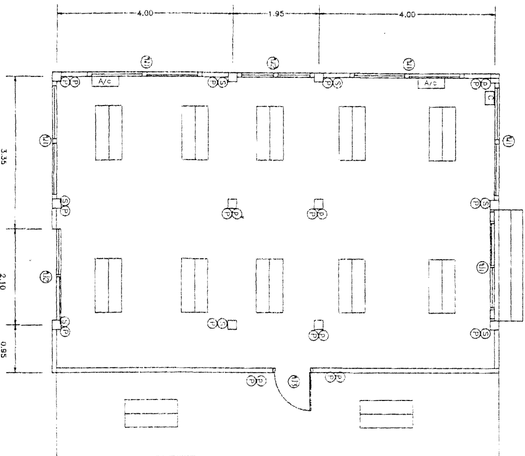
แผนผังไฟฟ้าห้องงานสารนิเทศชั้น ๒
