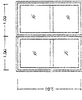
รูปที่ ๑-๒ บอร์ดบานเลื่อนบานกรอบไม้ยิปซัมกระจกใส ๒บานสูง ๒.๐๐ เมตร กว้างบานละ ๑.๐๐ เมตร กว้างบานละ ๑.๐๐ เมตร
